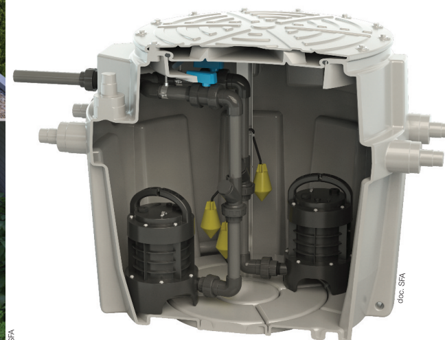
Station de relevage SANIFOS® 500 équipée de 2 pompes avec système de dilacération SFA.
